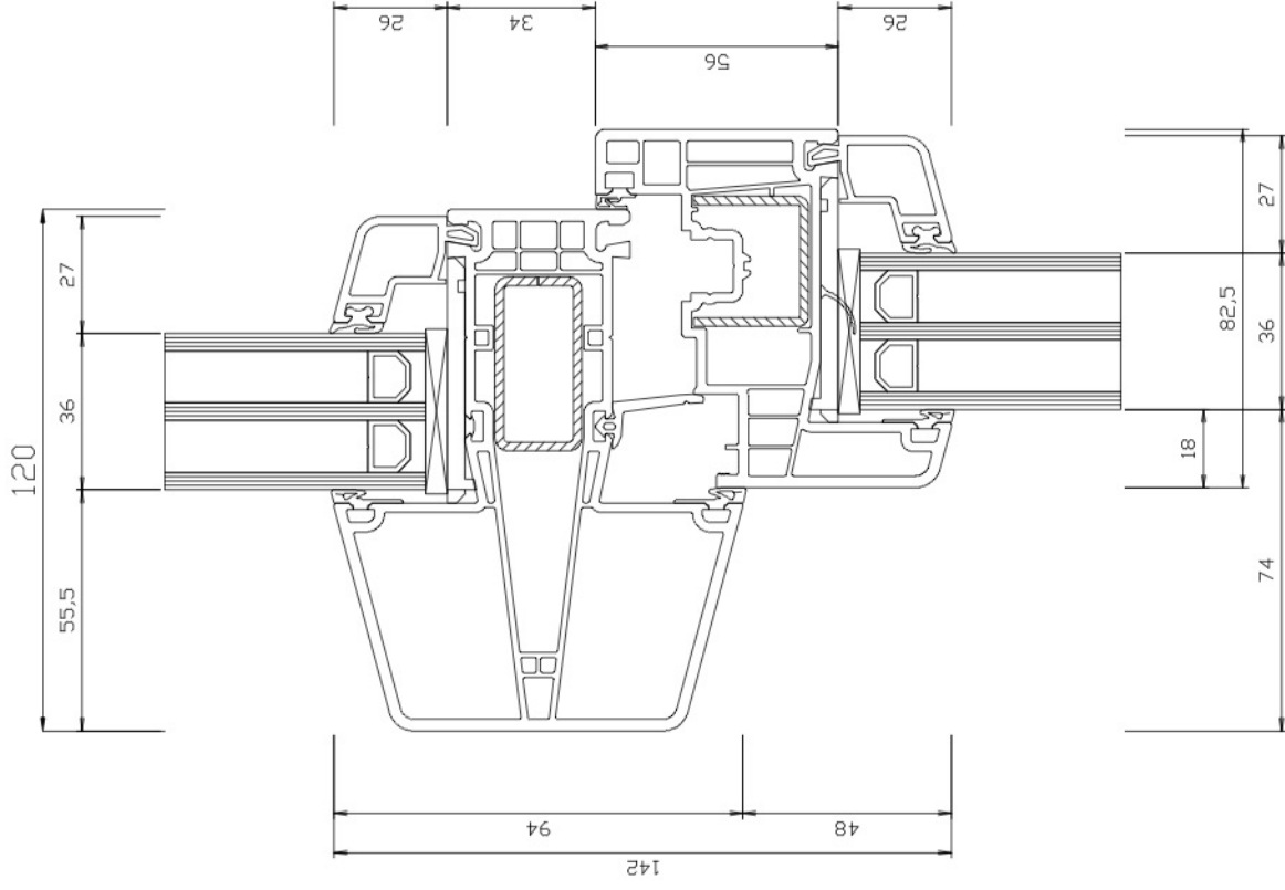
Detail: T1-A04-TD Schaal 1:2
